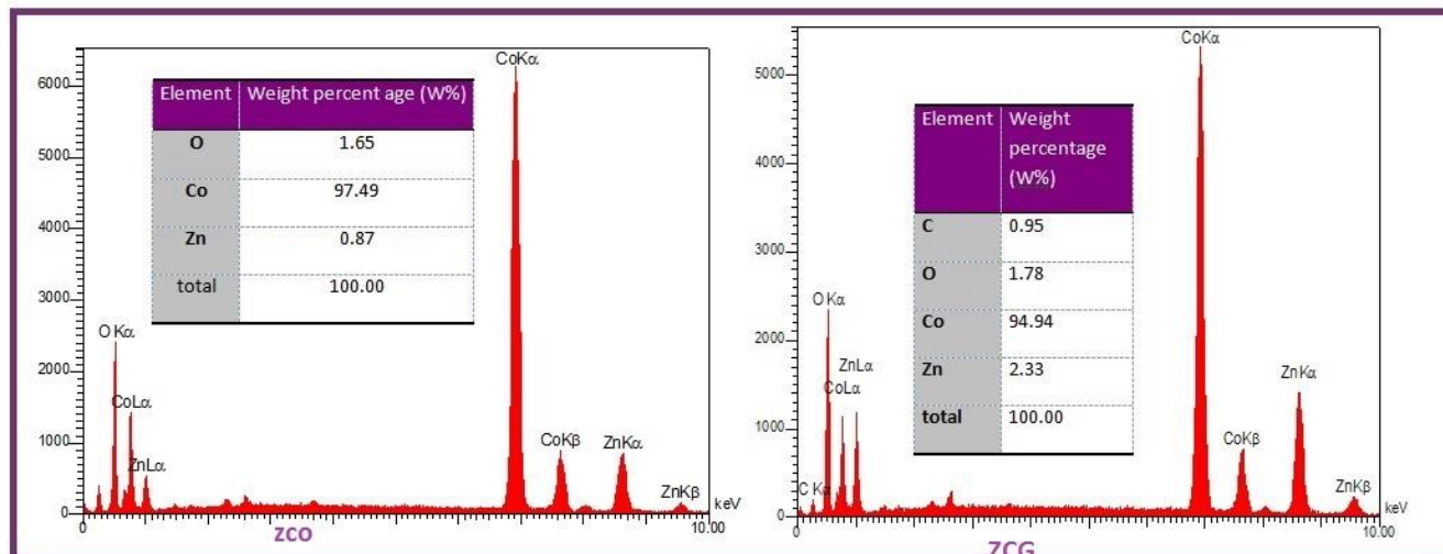
Fig. 5. EDS images of ZnCo_2O_4 (ZCO) and ZnCo_2O_4 /Graphene(ZCG)
