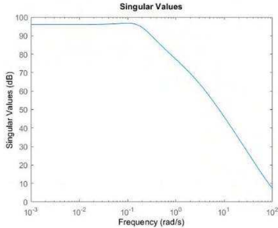
Fig. 3. Singular values
